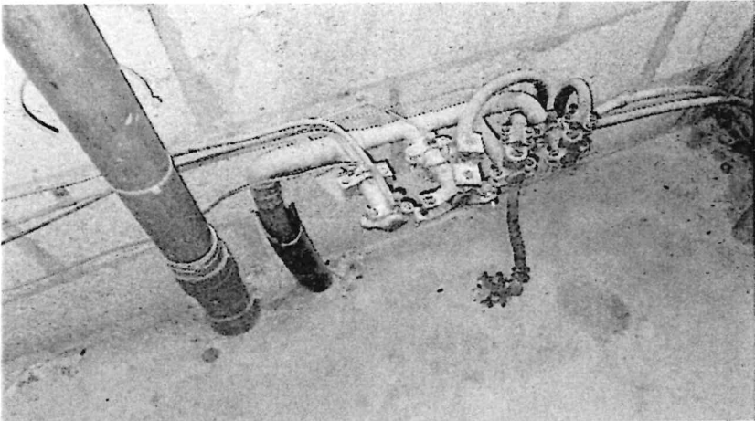
Conduits.
